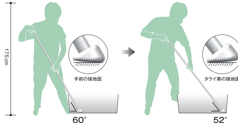
《 Type-L かい棒角度イメージ 》(手持ち棒部：1,350mm / 1.06kg +かい先 270g)
