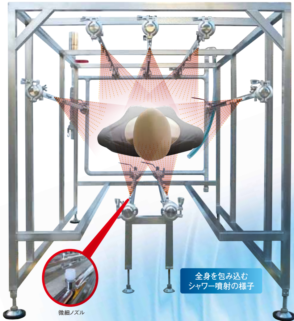
実際の作業時はシャワー飛散防止のため、カバーシートをかけて使用します。
